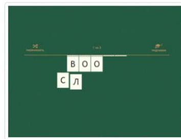
Криптон
