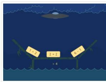
НЛО
